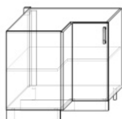
D/roh 78x78cm s deskou 90x90cm – skládaný
